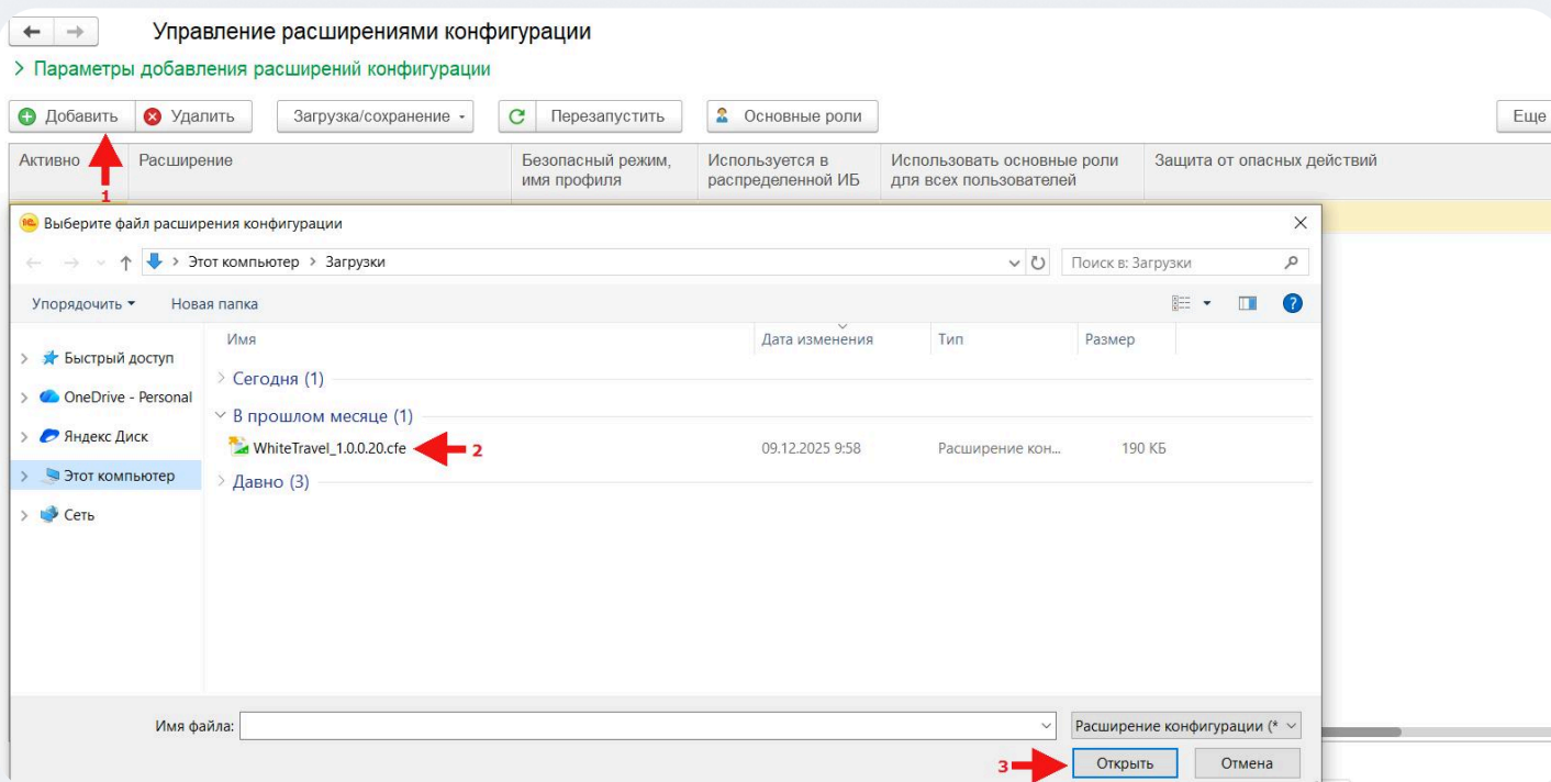
Добавление расширения конфигурации (обновленной версии)
